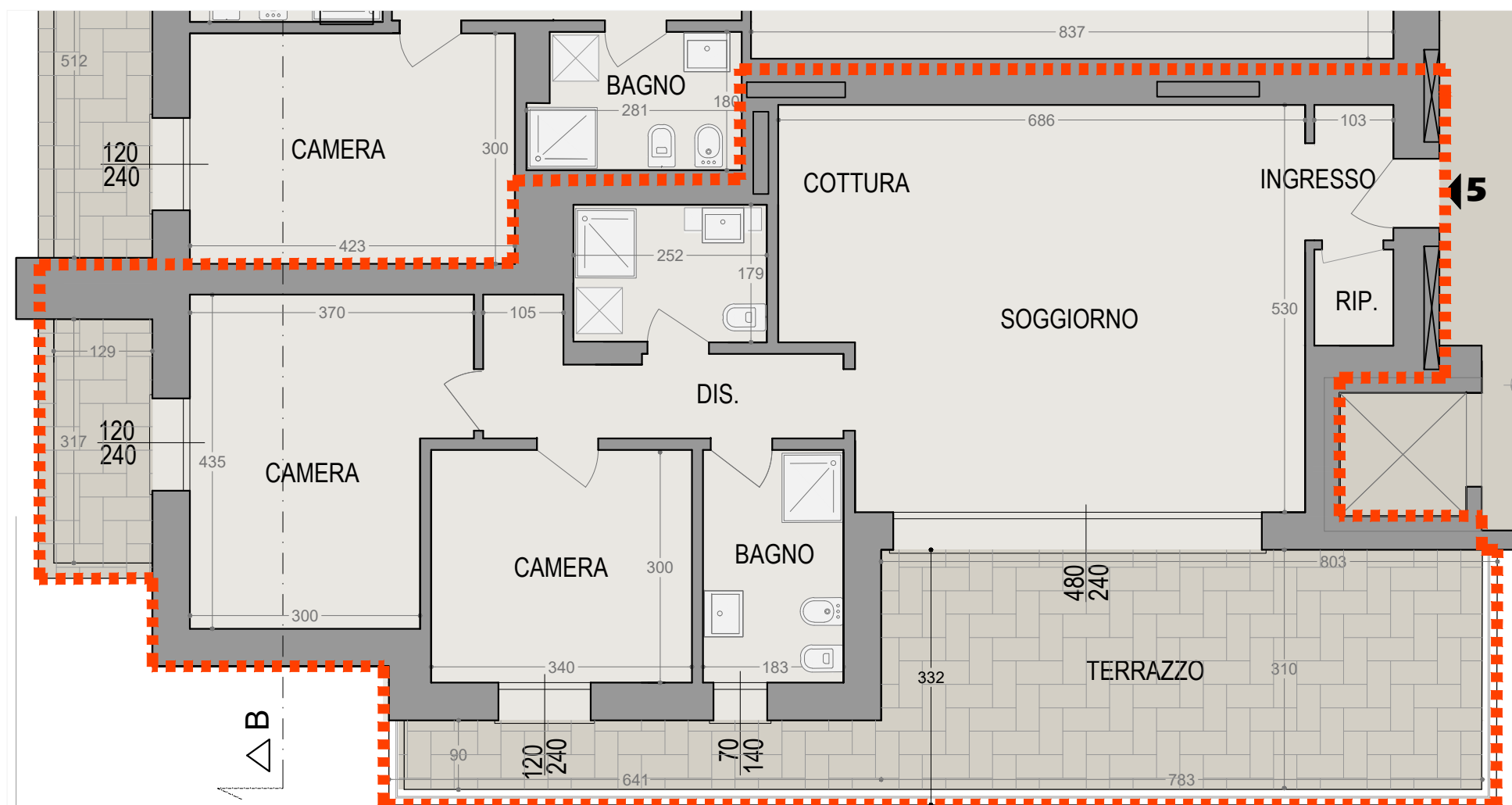
PIANO SECONDO - TIPOLOGIA TRILOCALE DOPPI SERVIZI
