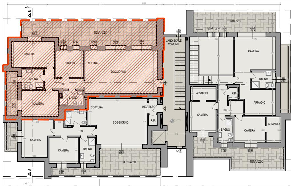
PLANIMETRIA GENERALE
