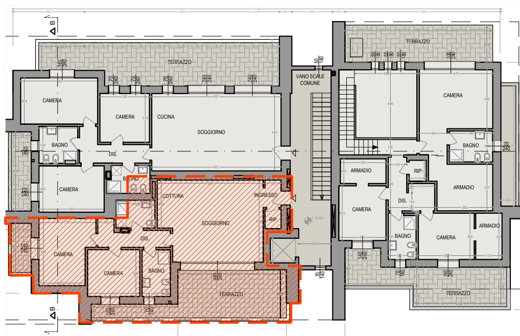
PLANIMETRIA GENERALE
