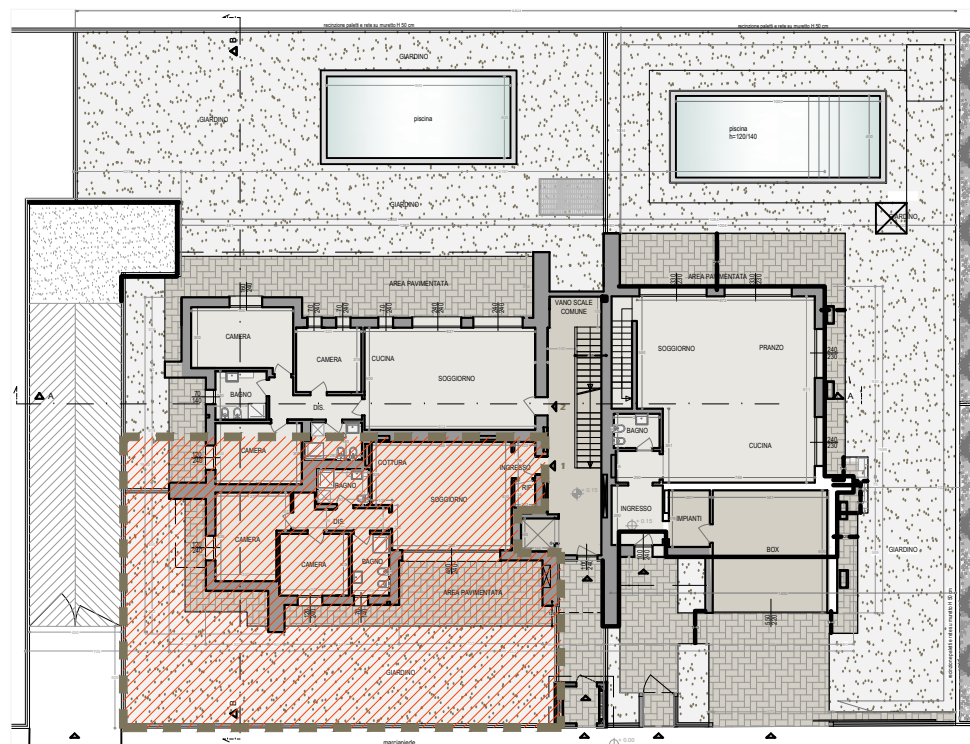
PLANIMETRIA GENERALE
